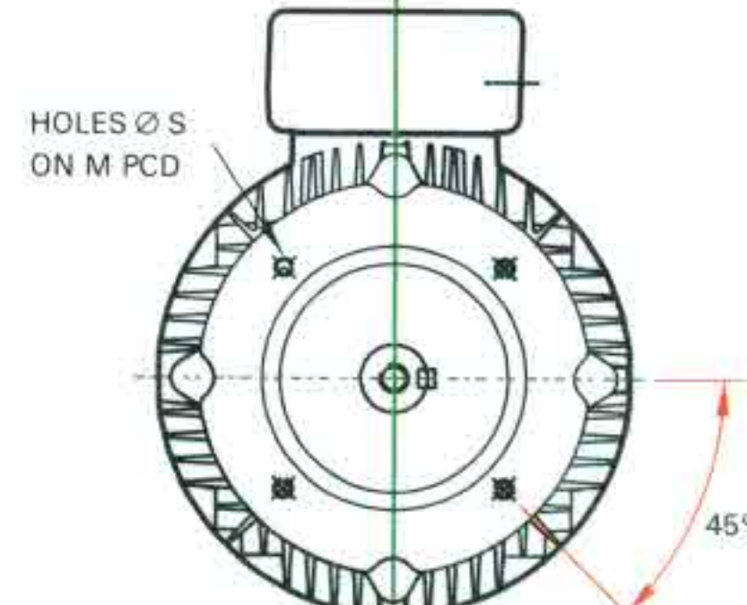
FACE MOUNTING IM - B14
