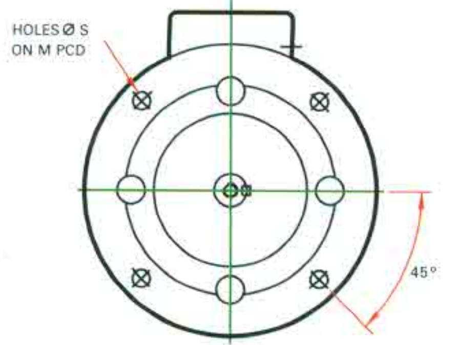
FLANGE MOUNTING IM - B5
